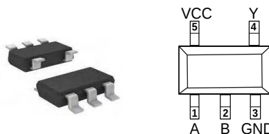
SOT23-5
