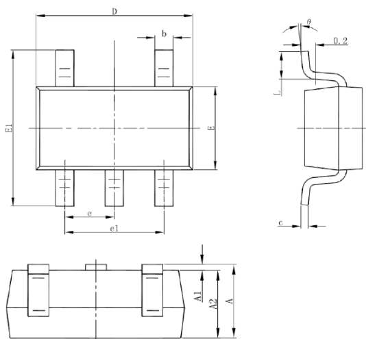
SOT-23-5L
