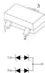
SOT-23
