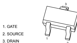
SOT-523
