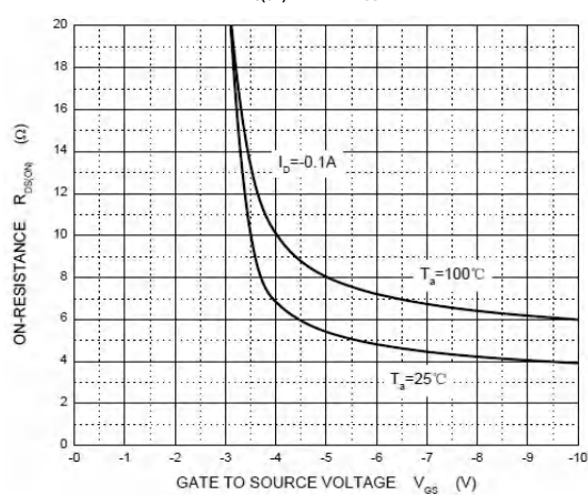
R_{DS(ON)} — V_{GS}
