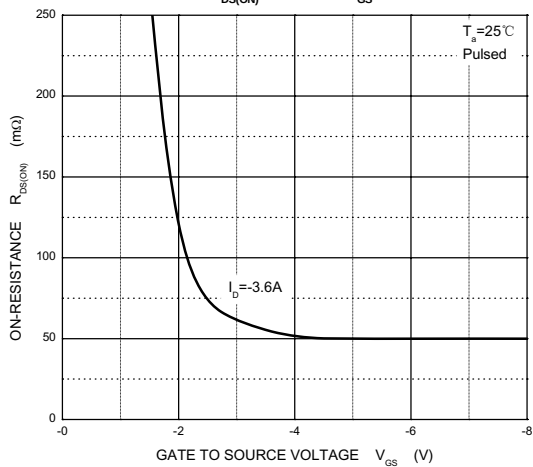
R_{DS(ON)} — V_{GS}
