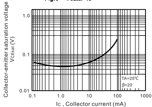
Fig.6 VCEsat--Ic
