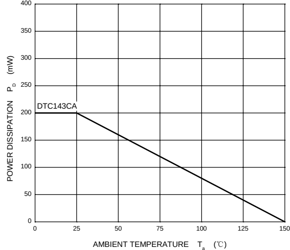
P_D — T_a
