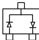
BAS70-04
