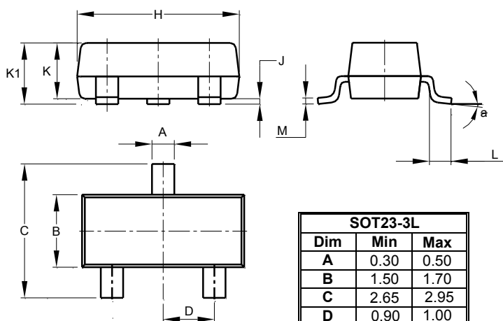
SOT23-3L
