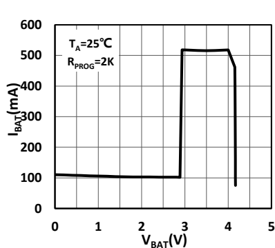
充电电流VS电池电压
