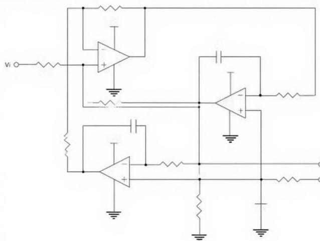
5 低漂移峰值检波器
