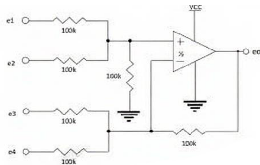
图 2 直流加法放大器
