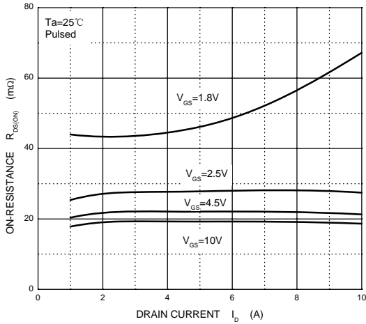
R_{DS(ON)} — I_D
